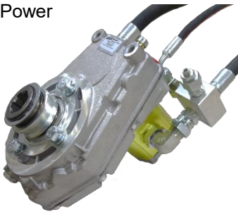
Hydr. lisäpumppu
