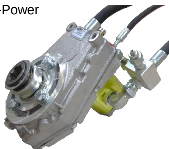
Hydr. lisäpumppu
